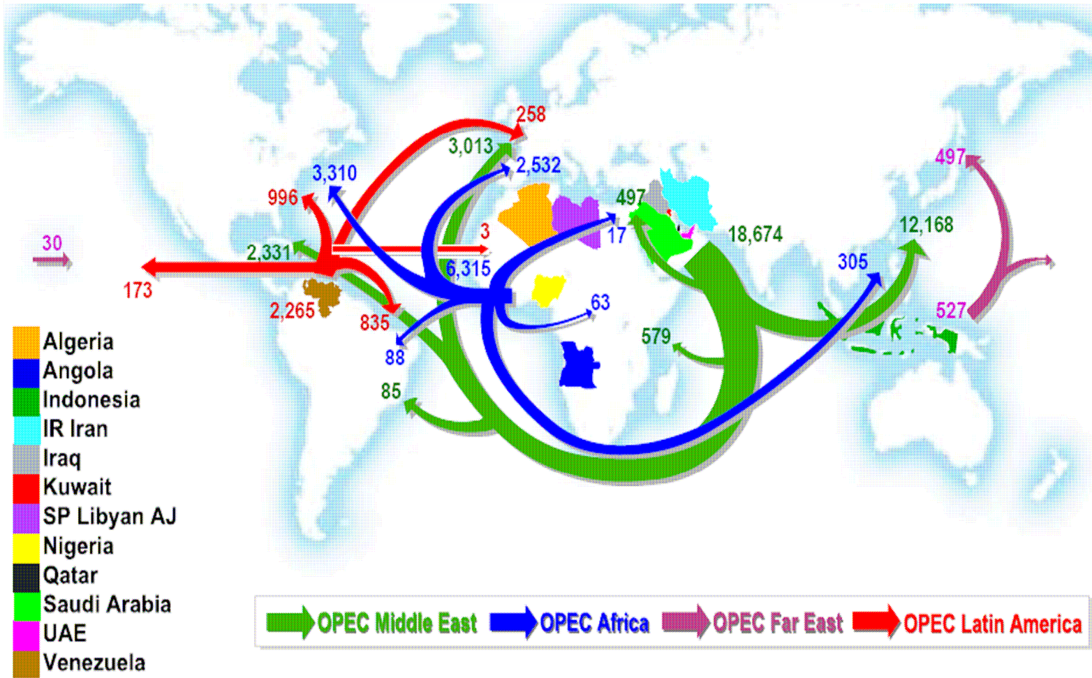
Figura 5 – Flussi di petrolio greggio e raffinato dai paesi OPEC (2006) - migliaia di barili al giorno -
