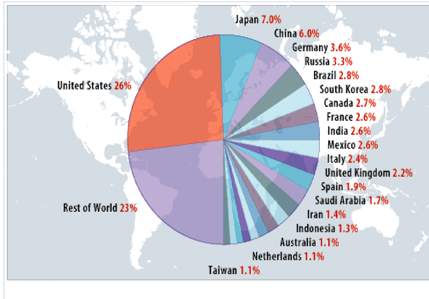
Figura 2 – Consumo mondiale di petrolio
