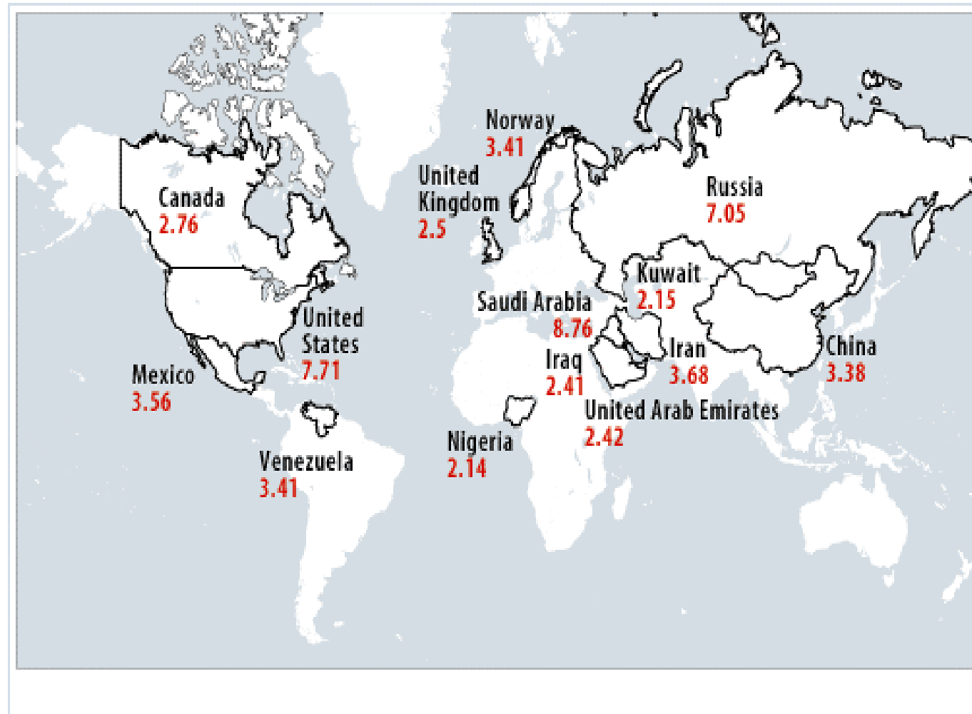
Figura 3 – Produzione mondiale di petrolio (milioni di barili al giorno)
