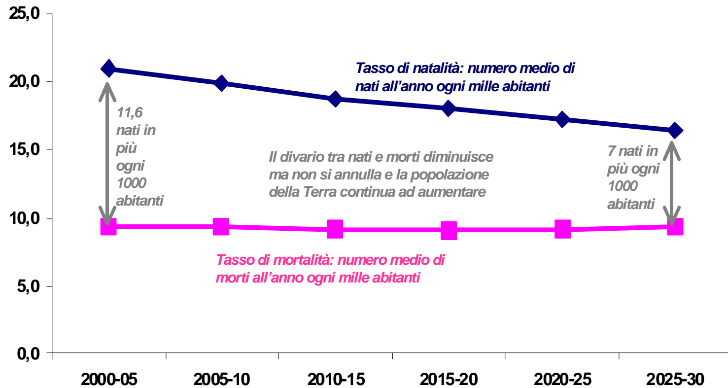
Figura 2 - Come si muoveranno la natalità e la mortalità
