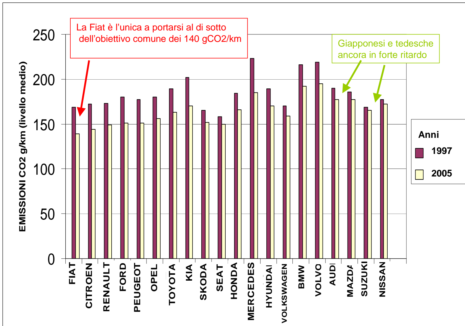
Figura 3: riduzione delle emissioni medie di CO2 per le principali case automobilistiche nel periodo 1997/2005
