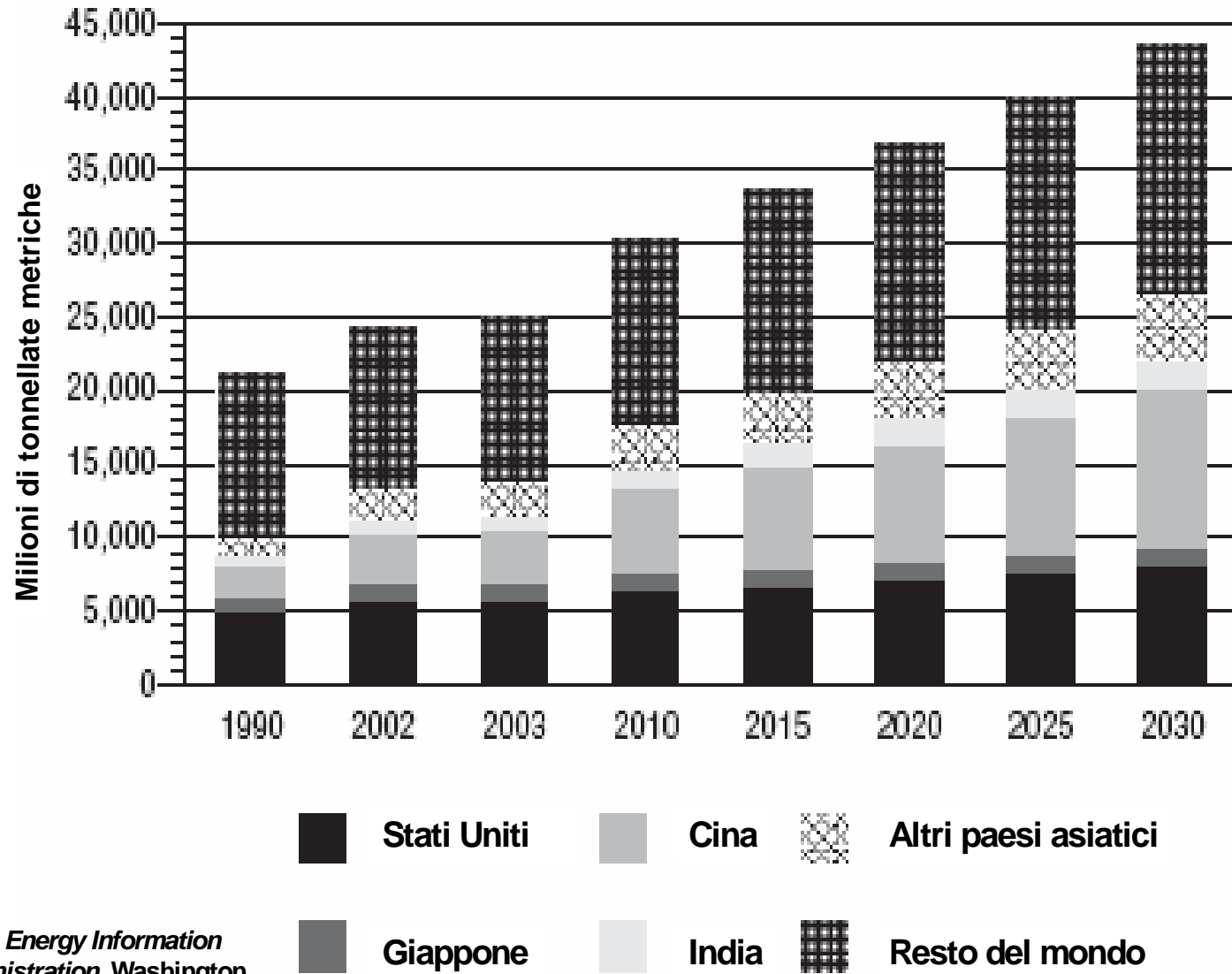
Figura 6: Emissioni mondiali di diossido di carbonio
